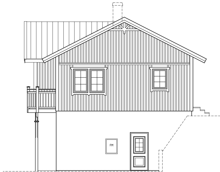
FASAD MOT
