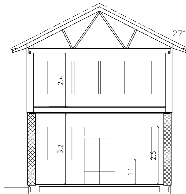
SEKTION C - C
