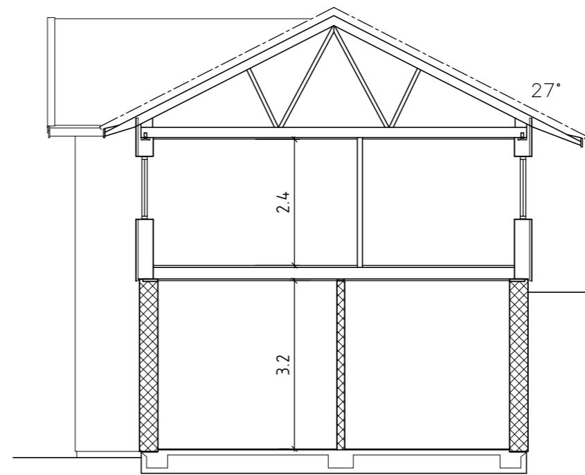
SEKTION B - B
