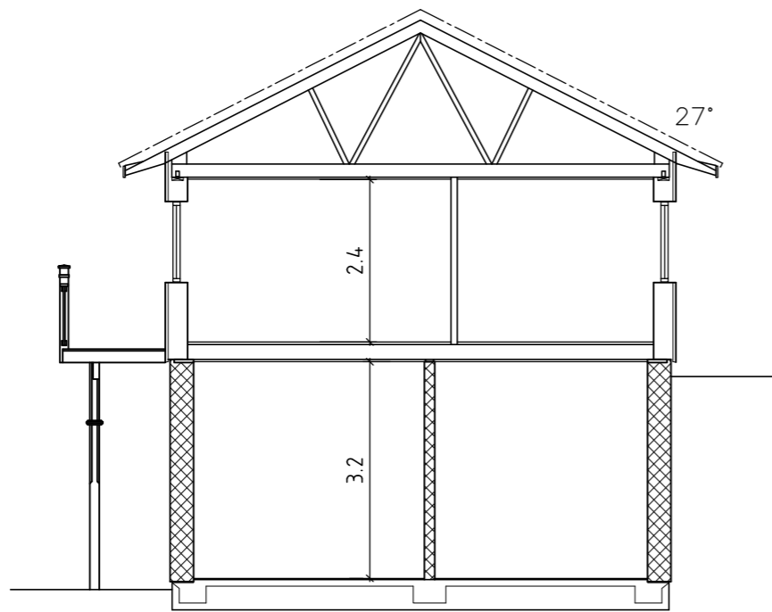
SEKTION A - A
